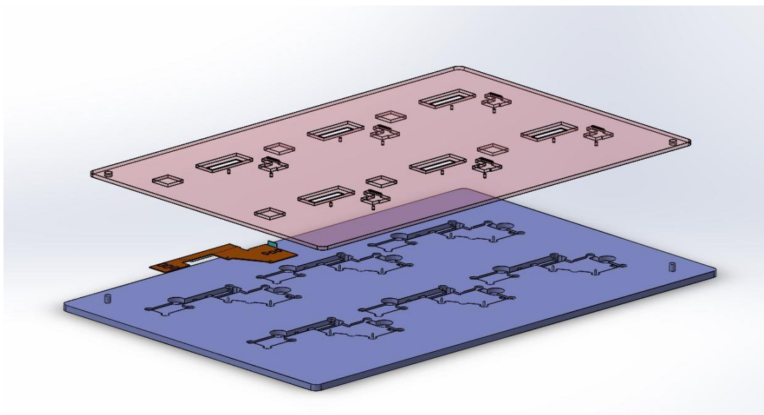
▲Soldering 新模具設計
